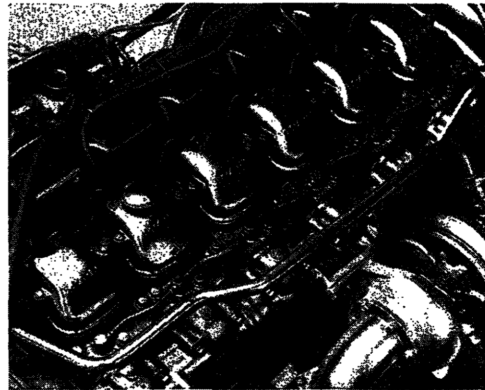
1985 M.A.N.-8-Zylinder-Reihomotor mit direkter Einspritzung und kombinierter Aufladung und Ladungshaltung, 350 PS Leistung, spezifischer Kraftstoffverbrauch im Optimum weniger als 200 g/kWh
